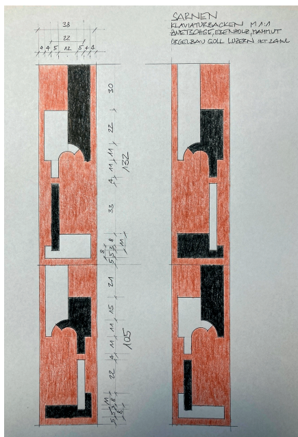
Entwurfszeichnung der Klaviaturbacken
